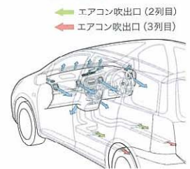
エアコン吹出口説明図
