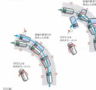
VSC説明図
