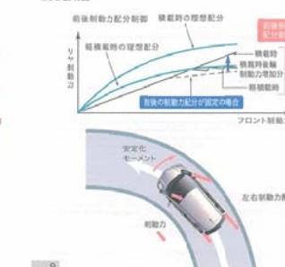
EBD説明図
