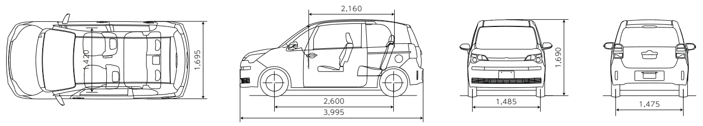
トヨタ スペイド 寸法図 F(2WD) 単位:mm
