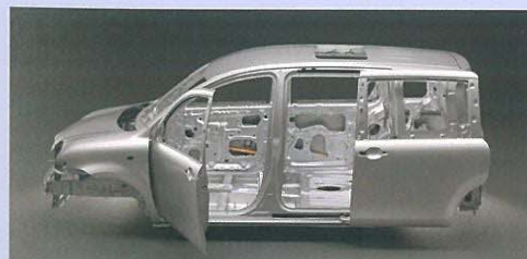
衝撃吸収ボディと高強度キャビン“GOA” ●写真のサイドアビームは機能説明のために着色したものです。
