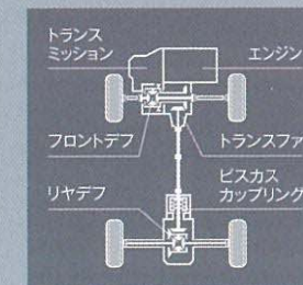
Vフレックスフルタイム4WDシステム図
