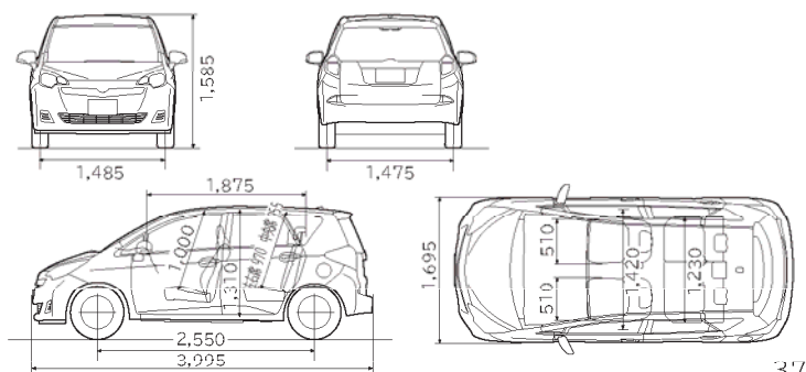
寸法図:トヨタラクティス 1.5G 2WD (単位:mm)
