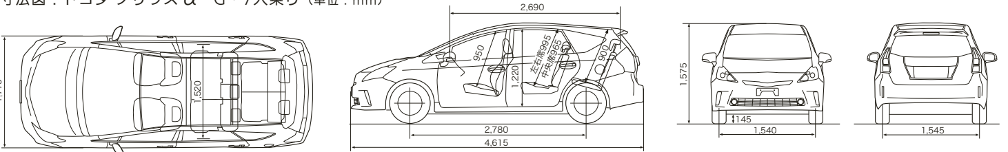
寸法図：トヨタ プリウス α G・7人乗り (単位：mm)
