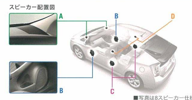
■写真は8スピーカー仕様。
