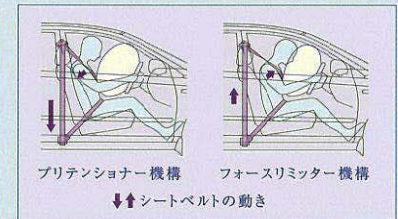
プリテンショナー&フォースリミッター機構説明図
