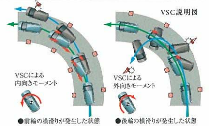
●前輪の横滑りが発生した状態
