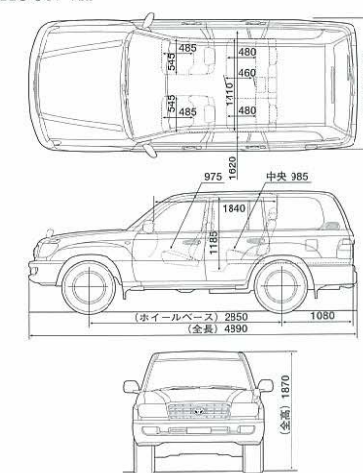
WAGON VX
