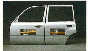
サイドドアビーム (説明のため着色したものです。)
