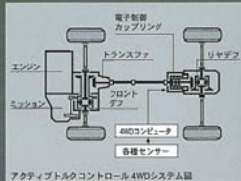
アクティブトルクコントロール4WDシステム図
