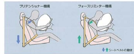
プリテンショナー&フォースリミッター説明図
