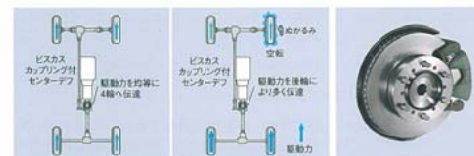
4WD (フルタイム4輪駆動方式)
