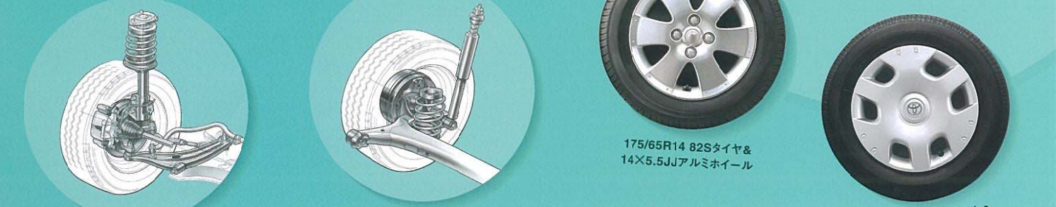
フロント:Lアーム式マックファーソンストラット式サスペンション リヤ:イータビームサスペンション(トーコレクト機能付トーションビームサスペンション)
