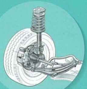
フロント: L-アーム式マックファーソンストラット式サスペンション
