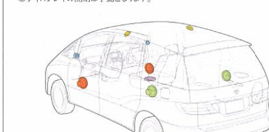
●16cmフロントフルレンジスピーカー ●12cmフロントウーファー (運転席下) ●3.5cmフロントツイーター ●6cmルーフフルレンジスピーカー ●14cmリヤフルレンジスピーカー
