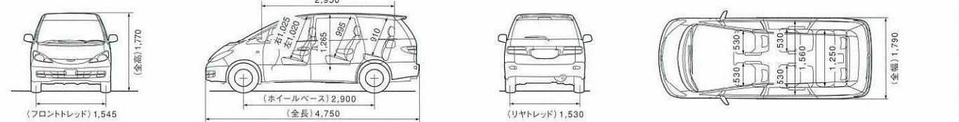
寸法図: G (3.0L / 7人乗り) 2WD <単位:mm>
