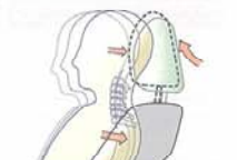
アクティブヘッドレスト作動イメージ
