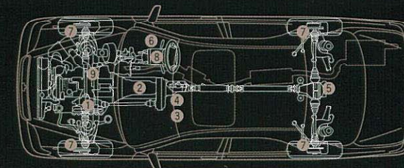
電子制御フルタイム4WDシステム図
