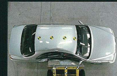
側面衝突実験 (55km/h、写真は実験用試作車です。)
