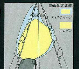
ディスチャージヘッドランプ (ロービーム) 配光図
