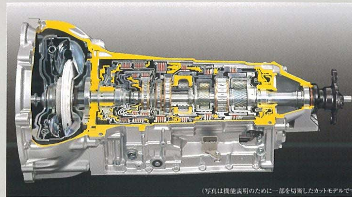
(写真は機能説明のために一部を切断了したカットモデルです)
