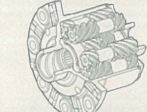
トルク感応型のリミテッドスリップデフ。左右輪の差動制限力により高速走行時の直進安定性を高め、また悪路での走破性も向上させます。
