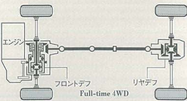
ビスカスカップリング式フルタイム4WD
