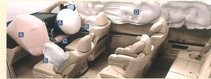
SRSエアバッグシステム: A SRSエアバッグ B SRSサイドエアバッグ C SRSニーエアバッグ D SRSカーテンシールドエアバッグ(左右)
